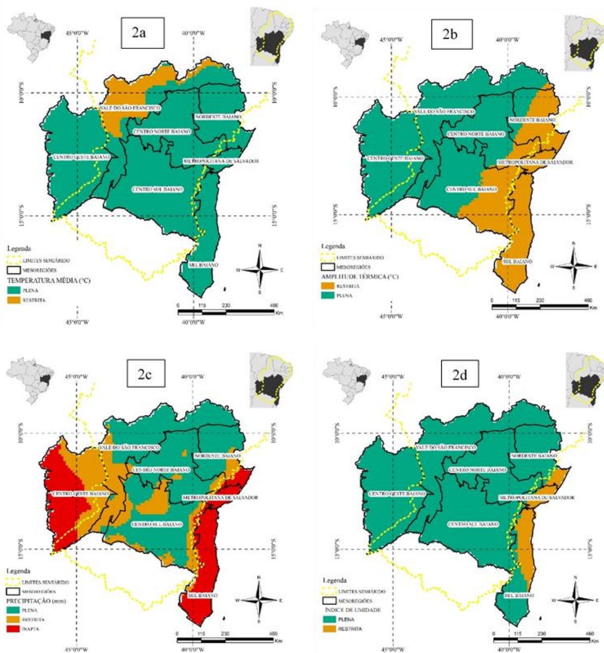
Figura 2. Mapas climatológicos anuais do estado da Bahia, Brasil: (a) Temperatura Média (°C), (b) Amplitude Térmica (°C), (c) Precipitação (mm) e (d) Índice de Umidade do Solo (adimensional).
